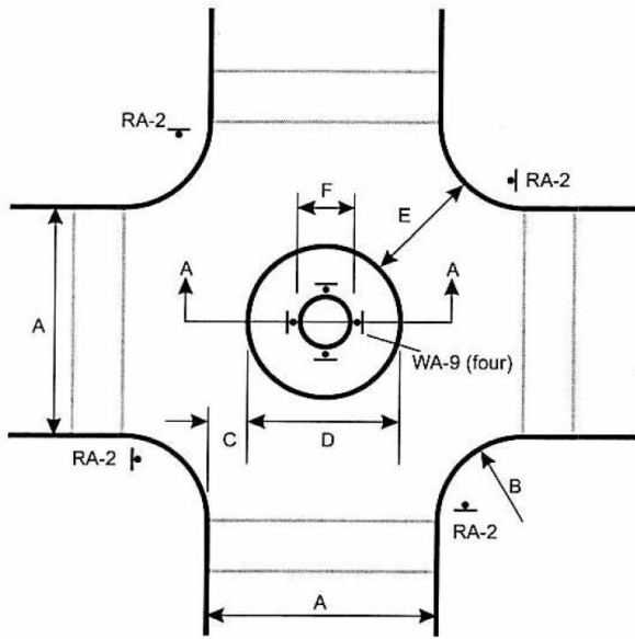
Figure 2.6 (7) Mini Traffic Circle
